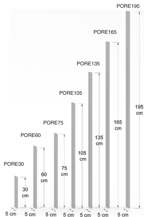
Poste remate p/ cambio de altura.
