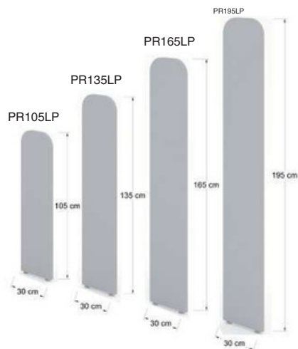
Poste remate con niveladores.
