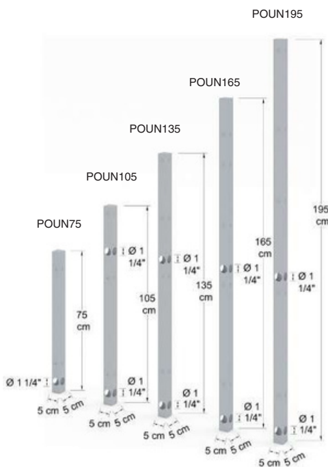
Poste unión en "L, T y cruceta".
