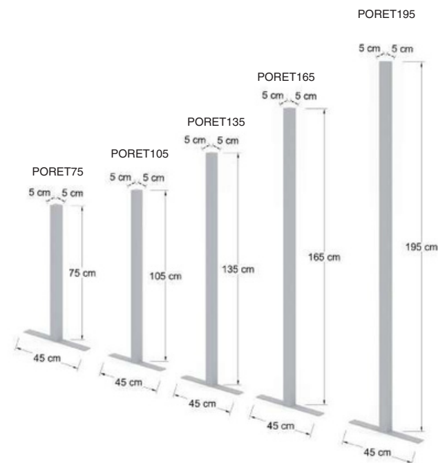
Poste remate en T para estabilizar mampara.
