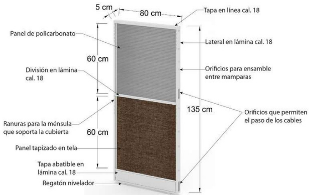
MAMPARA TAPIZADA CON POLICARBONATO PANEL SYSTEM I
