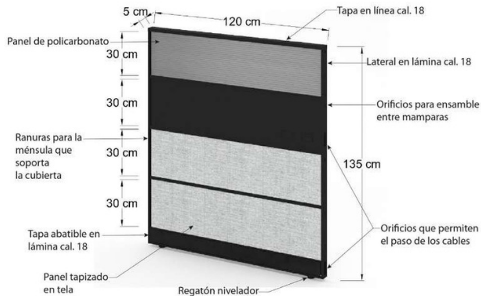
MAMPARA TAPIZADA CON POLICARBONATO PANEL SYSTEM III
