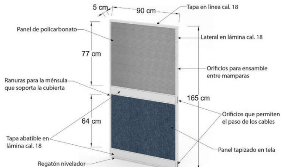
MAMPARA TAPIZADA CON POLICARBONATO PANEL SYSTEM II
