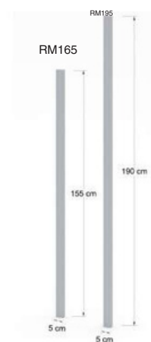
Remate de madera para fijar mampara a pared.
