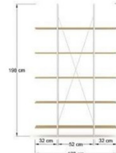
NS120 Librero de 5 entrepaños en mdf 15 mm., estructura metálica, tubular cuadrado de 3/4" y cruceta en redondo de 1/4".
