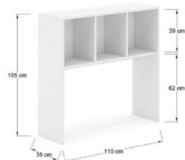
ALBR1035 Librero abierto fabricado en laminado plástico 19mm, con 3 nichos, sin forro en la parte baja. Para credenza de 120 cm.
