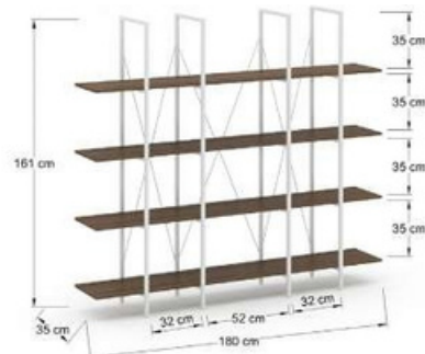
NS180 Librero de 4 entrepaños en mdf 15 mm., estructura metálica, tubular cuadrado de 3/4" y cruceta en redondo de 1/4".
