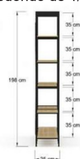
NS142 Librero de 4 entrepaños en mdf 15 mm., estructura metálica, tubular cuadrado de 3/4" y cruceta en redondo de 1/4".
