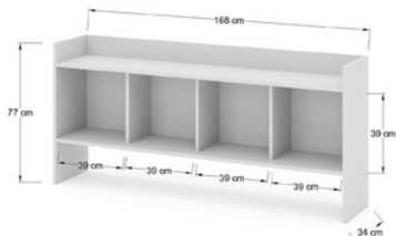
EXLB1634 Librero abierto fabricado en laminado plástico 19mm, con 4 nichos, sin forro en la parte baja.
