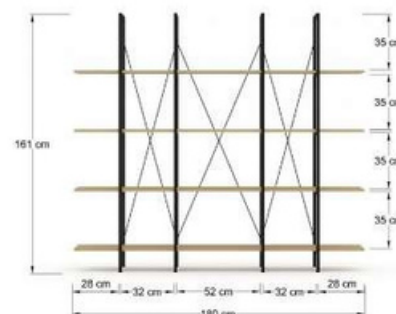
NS180 Librero de 4 entrepaños en mdf 15 mm., estructura metálica, tubular cuadrado de 3/4" y cruceta en redondo de 1/4".
