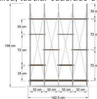
NS142 Librero de 4 entrepaños en mdf 15 mm., estructura metálica, tubular cuadrado de 3/4" y cruceta en redondo de 1/4".
