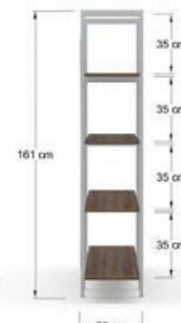
NS180 Librero de 4 entrepaños en mdf 15 mm., estructura metálica, tubular cuadrado de 3/4" y cruceta en redondo de 1/4".
