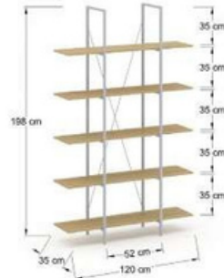
NS120 Librero de 5 entrepaños en mdf 15 mm., estructura metálica, tubular cuadrado de 3/4" y cruceta en redondo de 1/4".
