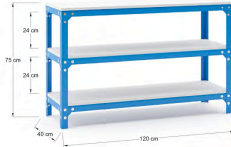
MECTV3-12 120 x 40 x 75
