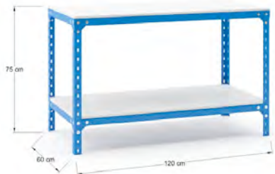
MECTV3-12 120 x 40 x 75
